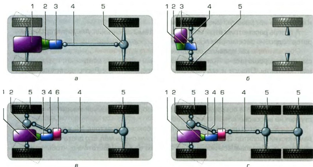
Рис. 26. Схемы трансмиссий автомобилей: а – заднеприводный автомобиль; б – переднеприводный автомобиль, в – полноприводный автомобиль колесной формулы 4х4; г – полноприводный автомобиль колесной формулы 6х6; 1 – двигатель; 2 – сцепление; 3 – коробка передач; 4 – карданная передача; 5 – ведущий мост; 6 – раздаточная коробка.
