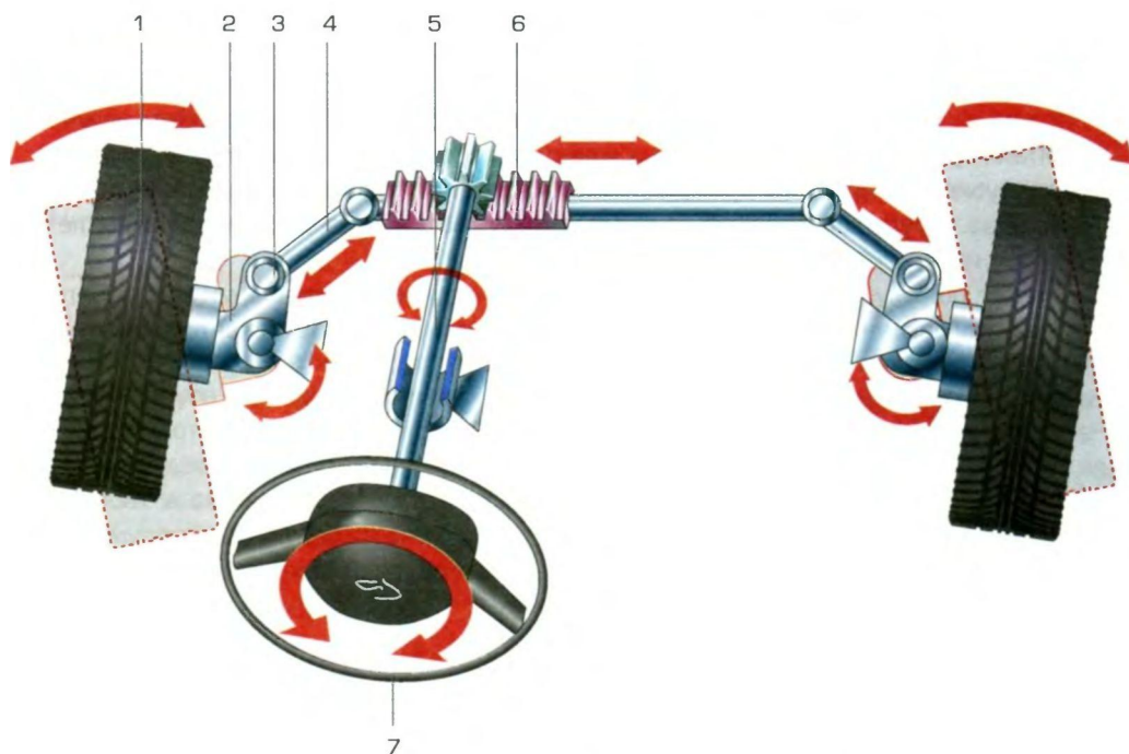
Рис. 49. Схема работы рулевого управления «шестерня-рейка»: 1—переднее колесо; 2 — поворотный рычаг; 3 — рулевой шарнир; 4 — рулевая тяга; 5 — рулевой вал с шестерней; 6 — рейка рулевого механизма; 7 — рулевое колесо.
